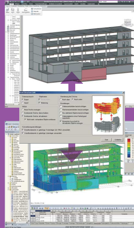
Statische Berechnung einer Schule in Laupheim. Mit freundlicher Genehmigung von Ingenieurbüro Rohmer GmbH und Dlubal
